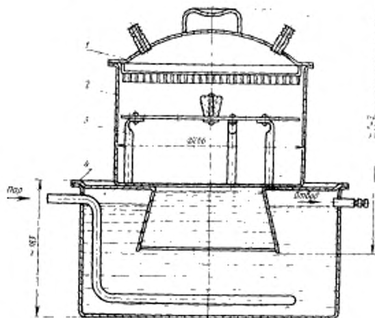
1—крышка; 2—корпус; 3—подставка с отверстиями для фильтров; 4—подъемная баня
