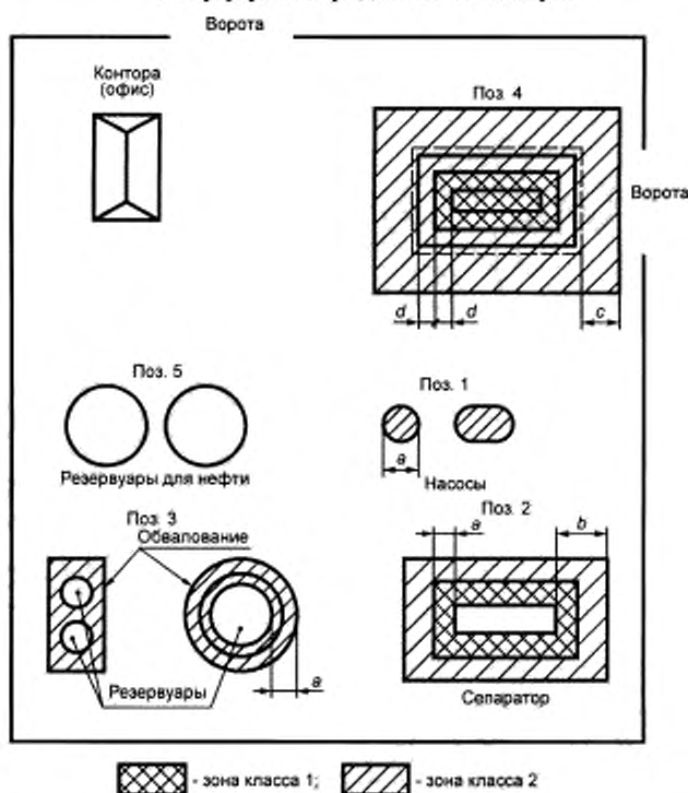
Пример № 11 Резервуарный парк для бензина и нефти
