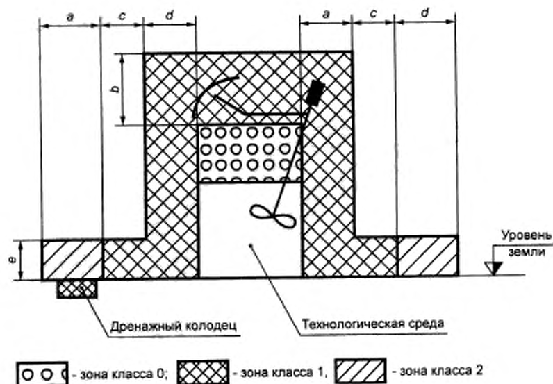
Пример № 5 Установленный внутри помещения резервуар, крышка которого периодически открывается. Горячая жидкость закачивается в резервуар и выкачивается из него через сварные трубопроводы, присоединенные к резервуару фланцами
