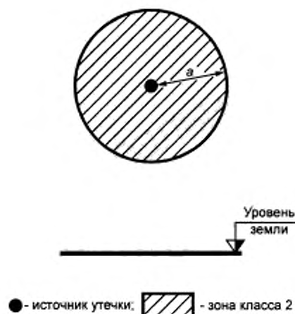
Пример № 4 Клапан сброса горячего газа, установленный на закрытом участке трубопровода
