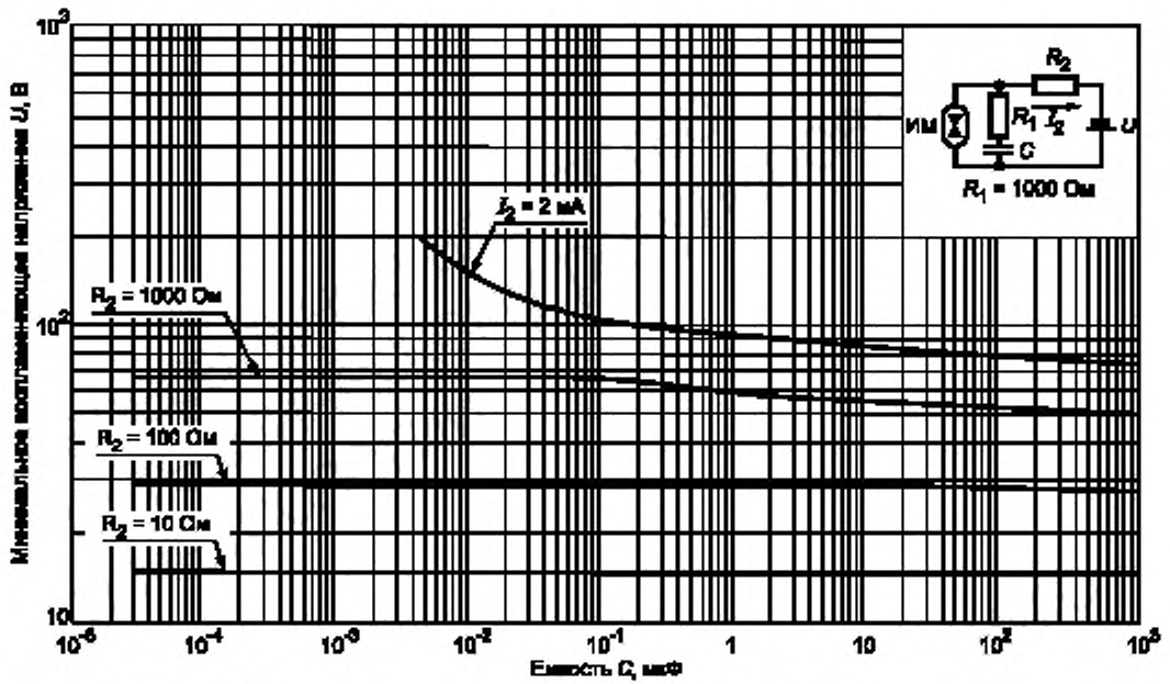
Рисунок А.19 — Минимальное воспламеняющее напряжение в активизированной взрывоопасной водородно-кислородной смеси (75 % H_2 + 25 % O_2 ) для емкостных цепей подгруппы ПВ при R_1 = 1000 \text{ Ом}
