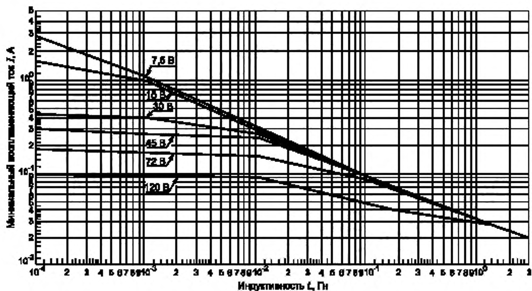
Рисунок А.8 — Индуктивные цепи подгруппы IIIA
