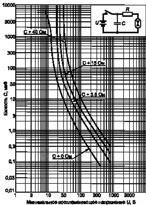
Рисунок А.2 — Емкостные цепи группы I
