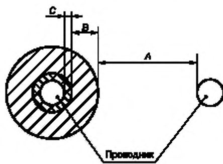
Рисунок В.5 — Измерение сложных расстояний
