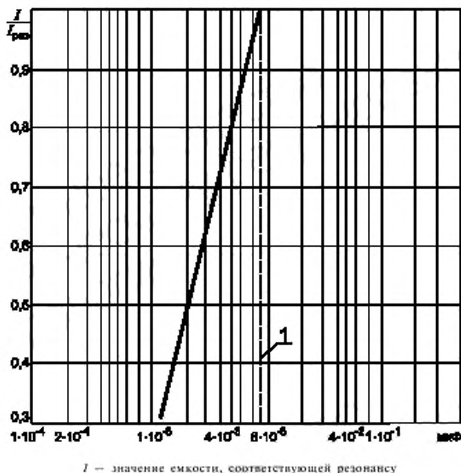
Рисунок А1.16— Зависимость снижения воспламеняющего тока ( I ) относительно воспламеняющего тока при резонансе ( I_{рез} ) от емкости при постоянных индуктивностях и частотах
