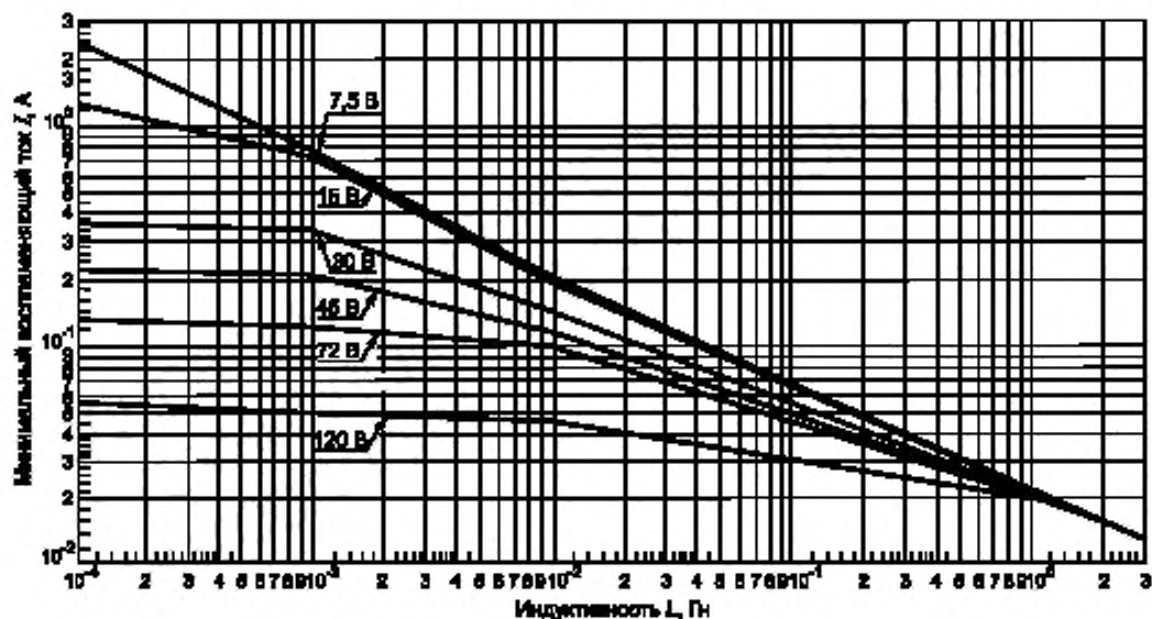
Рисунок А.9 — Индуктивные цепи подгруппы IIIB
