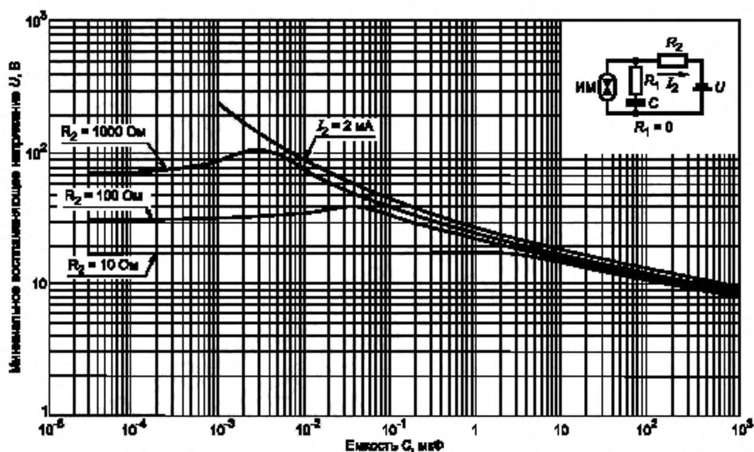
Рисунок А.12 — Минимальное воспламеняющее напряжение в активизированной взрывоопасной водородно-кислородной смеси (81 % H_2 + 19 % O_2 ) для емкостных цепей подгруппы ПА при R_1 = 0 \text{ Ом}
