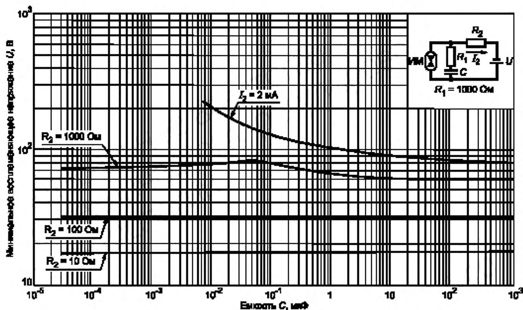
Рисунок А.15 — Минимальное воспламеняющее напряжение в активизированной взрывоопасной водородно-кислородной смеси (81 % H_2 + 19 % O_2 ) для емкостных цепей подгруппы ПА при R_1 = 1000 \text{ Ом}
