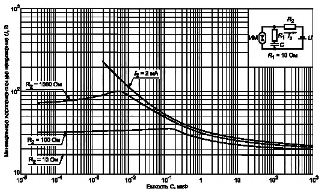
Рисунок А.13 — Минимальное воспламеняющее напряжение в активизированной взрывоопасной водородно-кислородной смеси (81 % H_2 + 19 % O_2 ) для емкостных цепей подгруппы IIIA при R_1 = 10 \text{ Ом}
