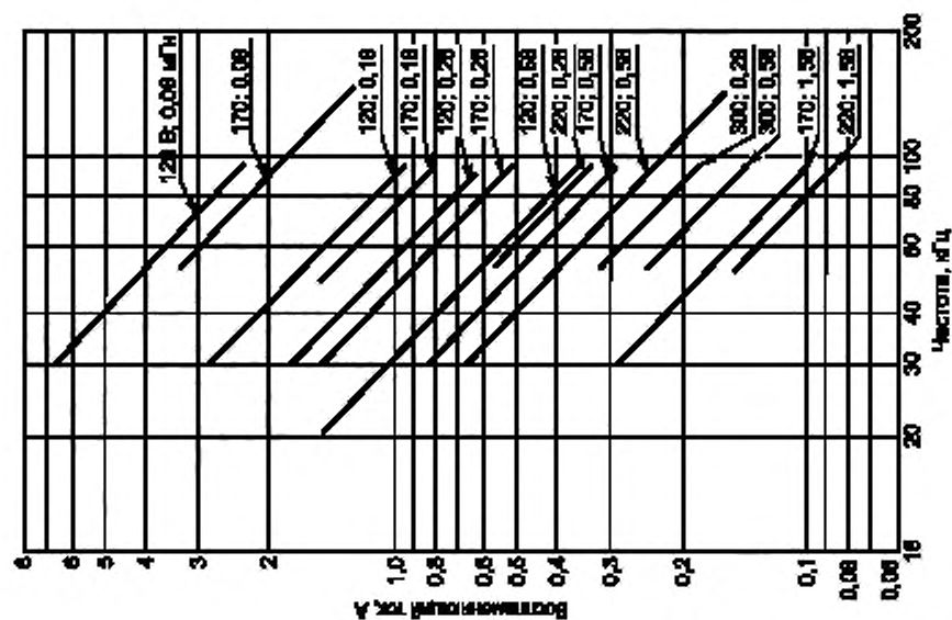
Рисунок А1.15— Зависимость воспламеняющего тока от частоты, индуктивнос- ти и напряжения источника для метановоздушной смеси
