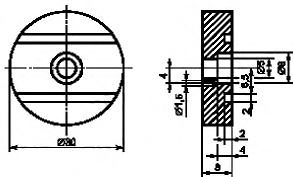
Рисунок Б.2 — Кадмиевый контактный диск
