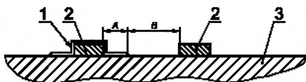
1 — лак; 2 — проводник; 3 — подложка
