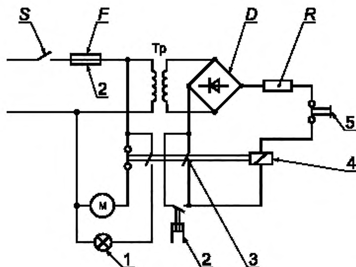
Рисунок Б.6 — Электрическая схема автоматической остановки работы взрывной камеры с помощью датчика давления
