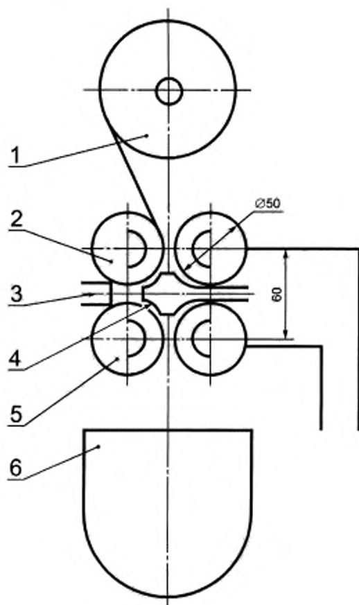
Рисунок Б.10 — Кинематическая схема искрообразующего механизма III типа
