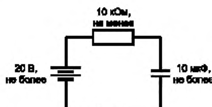
Рисунок А.24 — Простая емкостная цепь
