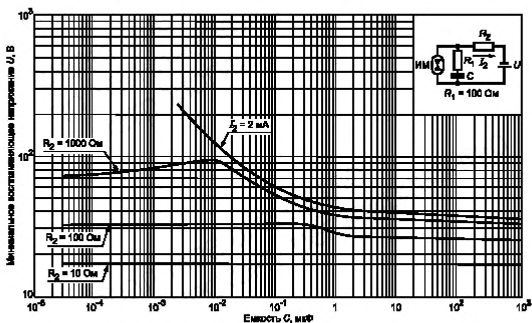
Рисунок А.14 — Минимальное воспламеняющее напряжение в активизированной взрывоопасной водородно-кислородной смеси (81 % H_2 + 19 % O_2 ) для емкостных цепей подгруппы IIIA при R_1 = 100 \text{ Ом}
