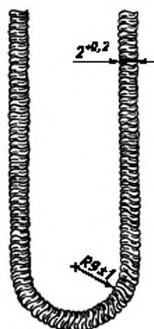
Рисунок Г.4 — Испытательная цепочка
