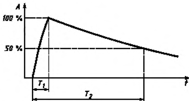
Рисунок Е.2 — Форма грозового импульса и импульса перенапряжения по линии связи
