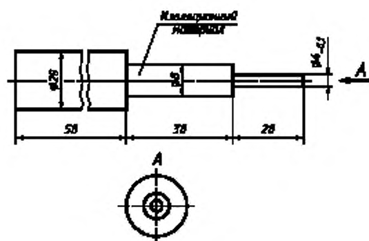
Рисунок Г.3 — Стандартный испытательный штырь
