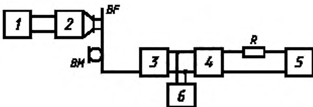
Рисунок Е.4 — Схема для измерения уровня звукового давления
