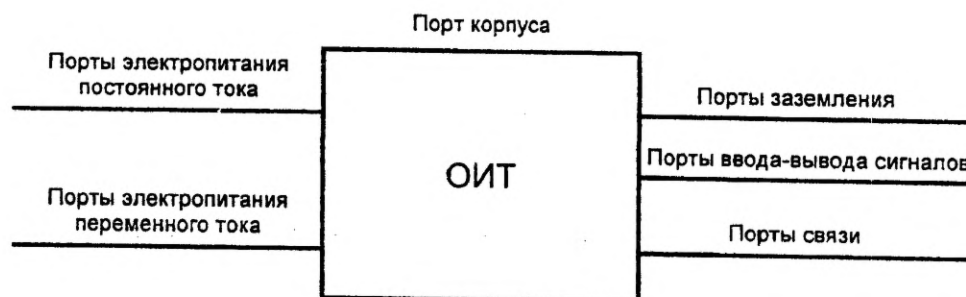
Рисунок 1 — Примеры портов ОИТ
