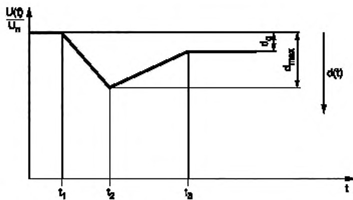
Рисунок 3 — Характеристика относительного изменения напряжения
