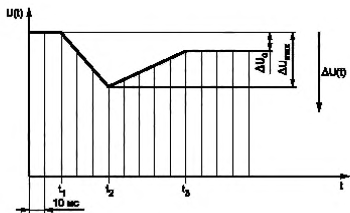
Рисунок 2 — Схема определения огибающей среднеквадратичных значений напряжения
