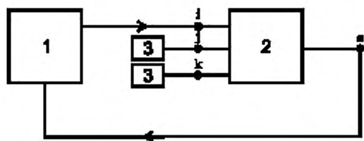
1 — измеритель комплексных коэффициентов передачи; 2 — устройство сложения; 3 — согласованные нагрузки; i, k — входы устройства сложения
