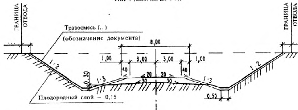
Тип 4 (выемка до 5 м)
