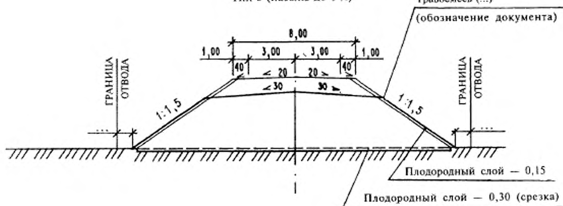
Тип 3 (насыпь до 6 м)
