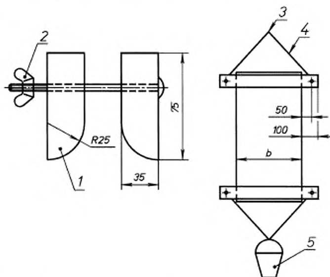
1 — зажим; 2 — крыльчатая гайка; 3 — точка подвеса; 4 — перевка; 5 — ведро с песком или захват разрывной машины
