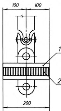
1 — плоская жесткая пластина; 2 — образец
