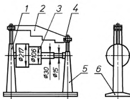
1 — опора; 2 — прижимная планка; 3 — цилиндр; 4 — гайка; 5 — опора; 6 — основание
