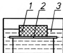
1 — образец; 2 — сетчатая подставка; 3 — ванна с водой
