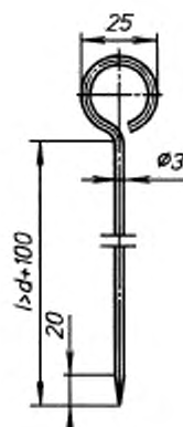
Рисунок А.2 — Игла
