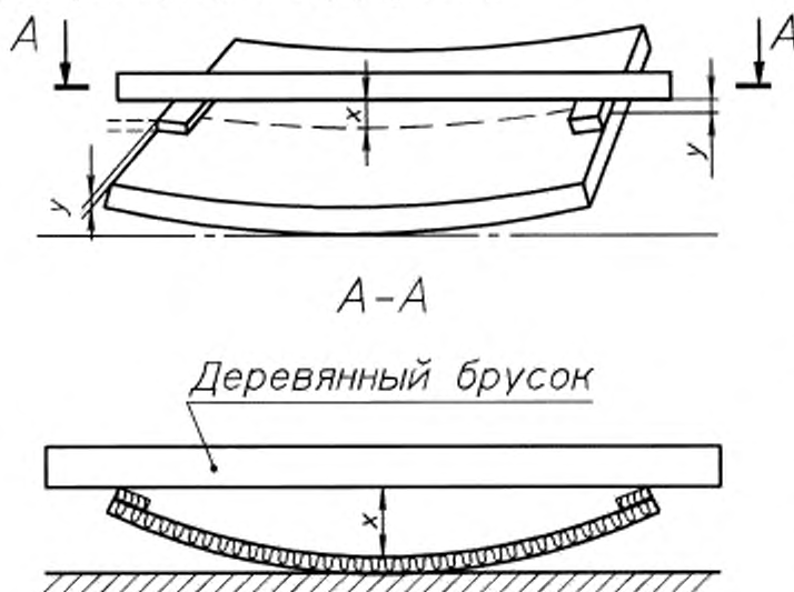
Рисунок Б.3 — Измерение отклонения от плоскостности плиты
