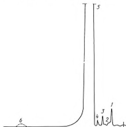
Типовая хроматограмма дифторхлорметана
