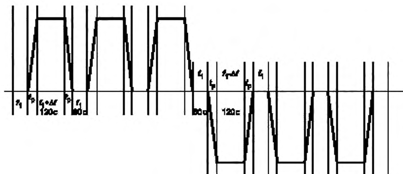
Рисунок 1 — Последовательность изменений частоты
