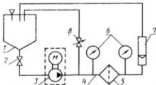
1 - расходный бак, 2, 8 - вентили; 3 - насос; 4 - соединительные трубы и впаивки; 5 - испытуемый фильтр; 6 - манометры; 7 - расходомер
