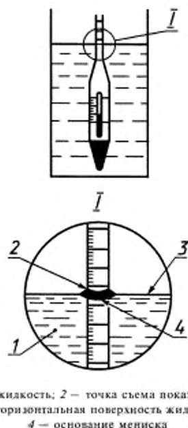
Рисунок 2 — Показание шкалы ареометра для непрозрачных жидкостей
