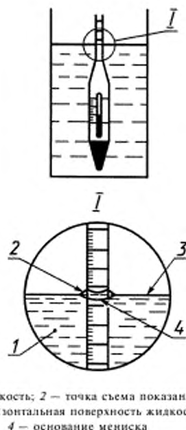
Рисунок 1 — Показание шкалы ареометра для прозрачных жидкостей
