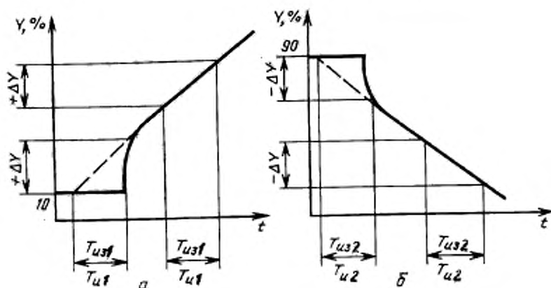
График для определения времени изодрома и интегрирования
