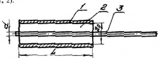
1 — оболочка; 2 — уплотненный порошок; 3 — стержень
