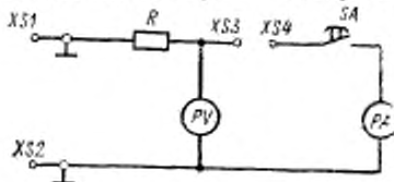
РА—амперметр; PV—вольтметр.
