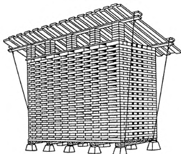
Составной штабель заготовок
