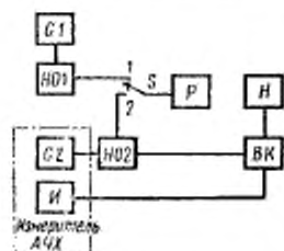
G1 — генератор стандартных сигналов; G2 — генератор качающейся частоты; P — измеритель частоты; S — переключатель; H01 , H02 — направленные ответвители; I — индикаторное устройство; BK — выходной контур; H — нагрузка
