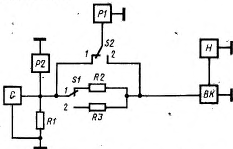
G—генератор стандартных сигналов (далее — генератор); R_1 —согласующий резистор; R_2 , R_3 —развязывающие резисторы; P_1 —измеритель уровня напряжений; P_2 —измеритель частоты; S_1 , S_2 —переключатели; BK—входной контур (система связанных контуров); H—нагрузка
