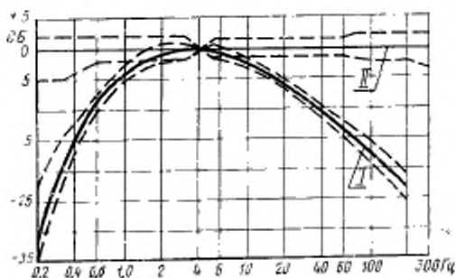
Частотные характеристики детонатора
