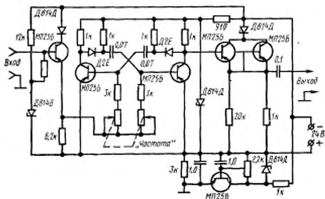
Принципиальная электрическая схема вспомогательного устройства
