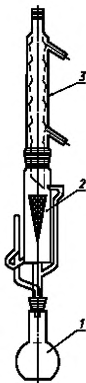
1 — колба; 2 — насадка; 3 — холодильник
