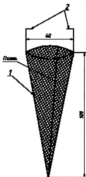
1 — сетка; 2 — держатели
