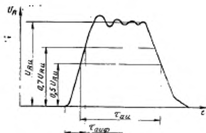
U_{Rn} — напряжение на измерительном резисторе в импульсе; \tau_{ан} — длительность импульса тока анода; \tau_{анф} — длительность фронта тока анода в импульсе
