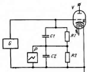
C_1, C_2 — конденсаторы делителя напряжения; G — источник импульсного напряжения; P — осциллограф; R_1, R_2 — резисторы делителя напряжения; V — испытываемый тиратрон
