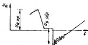
U_{a.пр} — прямое напряжение анода тиатрона; U_{a.обр} — обратное напряжение анода тиатрона Черт. 20
