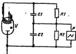
C1, C2 — конденсаторы делителя напряжения; P — осциллограф; R1, R2 — резисторы делителя напряжения; V — испытываемый газотрон Черт. 23
