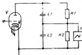
C1, C2 — конденсаторы делителя; P — осциллограф; R1, R2 — резисторы делителя; V — испытываемый тиатрон Черт. 19
