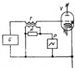
Г — источник импульсного напряжения; P — осциллограф; T — измерительный трансформатор тока; R — резистор; V — испытываемый тиратрон
