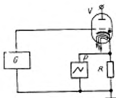
Г — источник импульсного напряжения; P — осциллограф; R — измерительный резистор; V — испытываемый тиратрон
