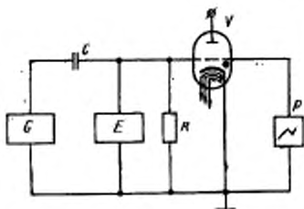
C — переходной конденсатор; E — фильтр; G — источник импульсного напряжения; P — осциллограф; R — резистор утечки; V — испытываемый тиристор
