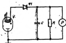
C — конденсатор; P — измеритель напряжения; R — резистор; VI — диод; V — испытываемый газотрон Черт. 22
