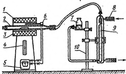
1—трубчатая печь; 2—кварцевая трубка; 3—лодочка; 4—рестат; 5—гальванометр; 6—термопара; 7—уравнительный сосуд, заполненный подкрашенной водой; 8—холодная вода; 9—мерная бюретка; 10—штатив
