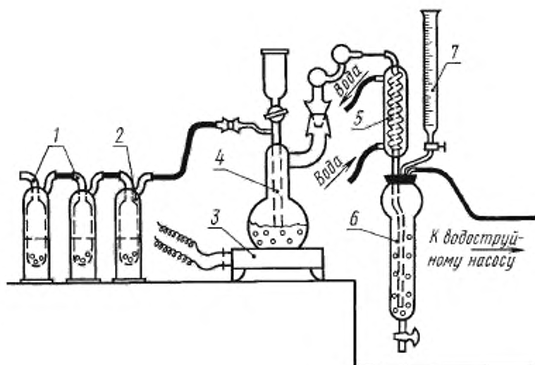
1 — склянка-ловушка с серной кислотой; 2 — склянка-ловушка с водой; 3 — электролитка; 4 — дистилляционная колба типа Кьельдаля из термостойкого стекла вместимостью 500 см 3 с пришлифованной пробкой, снабженной капельной воронкой с краном; 5 — холодильник; 6 — сосуд для улавливания аммиака; 7 — микробюретка
