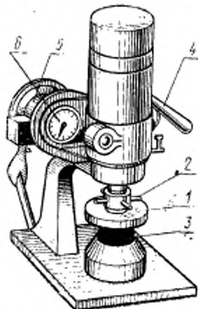
1 — патрон, 2 — гайка; 3 — подушка, 4 — щетка, 5 — мотор; 6 — шкала.
