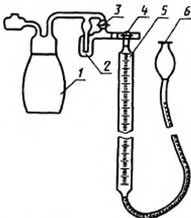
Прибор для определения массовой доли воды
