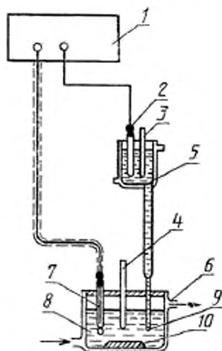
Схема измерения потенциала электрода
