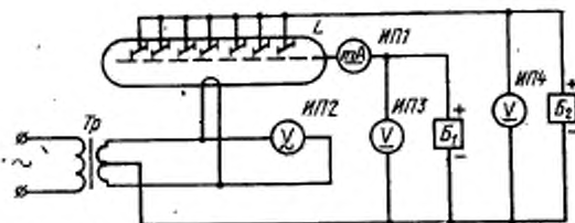
Б 1 , Б 2 —источники постоянного напряжения; ИП1—миллиамперметр; ИП2—вольтметр переменного напряжения; ИП3, ИП4—вольтметры постоянного напряжения; L—индикатор; Tr—трансформатор с выводом от средней точки обмотки накала
