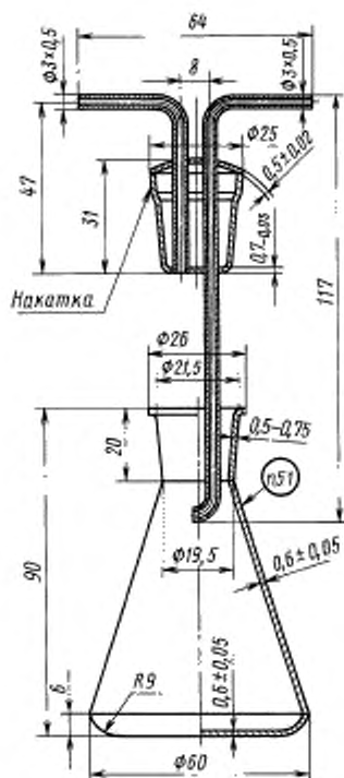
Приборы из платины для определения закиси железа Изделие № 419
