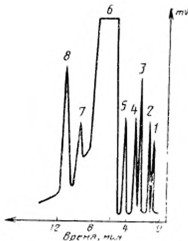
Типовая хроматограмма примесей в метилметакрилате
