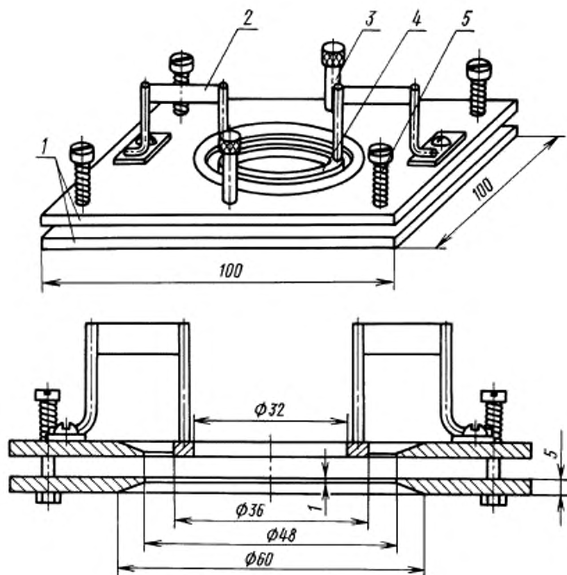
Трафарет для нанесения электродов
