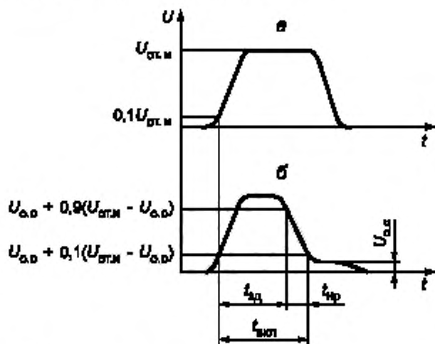
a — форма напряжения на выходе генератора G1 при отсутствии испытуемого тиристора; b — форма напряжения на испытуемом тиристоре; U_{о.о} — постоянное напряжение в открытом состоянии тиристора; U_{от.м} — импульсное отпирающее напряжение тиристора
