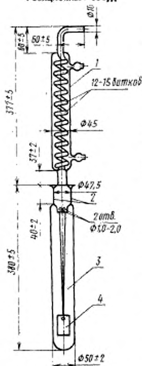
Реакционный сосуд
