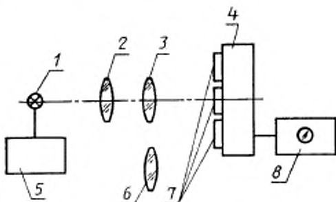
1 — источник света; 2 — коллиimator; 3 — эталонная насадка; 4 — фотоэлектрический колориметр; 5 — стабилизатор напряжения; 6 — испытуемая насадка; 7 — смешивные светофильтры; 8 — измерительный прибор
