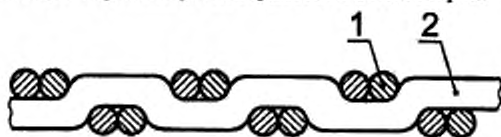
1 — нить основы ворсованная, 2 — нить утка ворсованная
