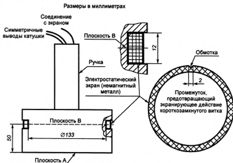
Рисунок А.1 — Конструкция рамочного датчика
