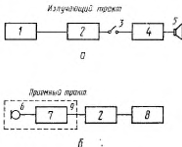
Блок-схема аппаратуры для измерения времени реверберации
