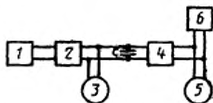
1 — низкочастотный генератор сигналов (н. 1.21); 2 — усилитель мощности (при необходимости); 3 — конденсатор с емкостью, равной емкости капсюля; 4 — ПУ — предварительный усилитель микрофона; 5, 5' — вольтметр (н. 1.4) (при необходимости); 6 — анализатор спектра (н. 1.5)
