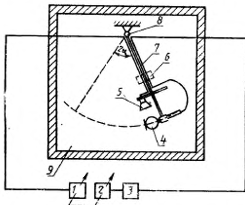
1 — низкочастотный генератор сигналов (п. 1.2.1); 2 — анализатор спектра (п. 1.5); 3 — самописец уровня (п. 1.2); 4 — испытуемый микрофон; 5 — указатель (п. 1.11.2); 6 — инерционная масса; 7 — кронштейн; 8 — горизонтальная ось; 9 — звукомерная заглушенная камера (п. 1.18)
