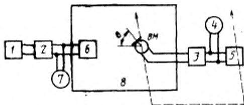
1 — низкочастотный генератор сигналов (п. 1.2.1) (или низкочастотный генератор шумовых сигналов (п. 1.2.2) — третьоктавный фильтр) (п. 1.8); 2 — усилитель мощности; 3 — измерительный усилитель (п. 1.3); 4, 7 — вольтметры (п. 1.4); 5 — установка для автоматической записи диаграммы направленности (п. 1.14); 6 — излучатель (п. 1.11.2); ВМ — испытуемый микрофон; 8 — помещение, обеспечивающее условия свободного поля (п. 2.3.1)
