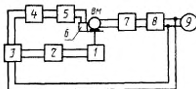
1 — вибростенд (п. 1.24); 2 — усилитель мощности (по необходимости); 3 — установка УАЗЧХ (п. 1.2); 4 — устройство автоматического регулирования (п. 1.11.1); 5, 7 — измерительные усилители (по необходимости) (п. 1.3); 6 — вибродатчик (п. 1.25); ВМ — испытуемый микрофон; 8 — сопровождающий избирательный фильтр (п. 1.9); 9 — вольтметр (п. 1.4)
