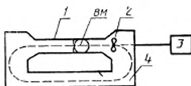
1 — рабочая часть; 2 — дощочки вентилятора; 3 — электрический двигатель; 4 — устройство «аэродинамическая труба»; ВМ — испытуемый микрофон
