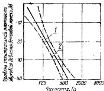
1 — теоретическое значение уровня спектральной плотности звукового давления ветровой помехи; 2 — границы допустимых отклонений
