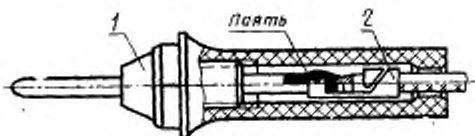
1—штыреволь; 2—наконечник
