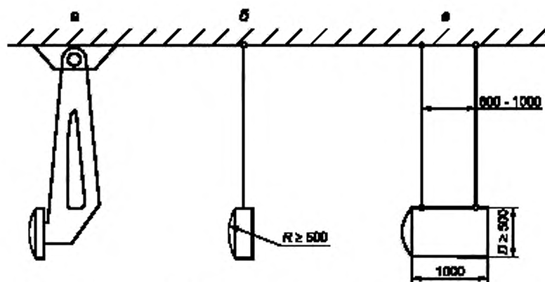
Рисунок 4 — Схема закрепления маятника
