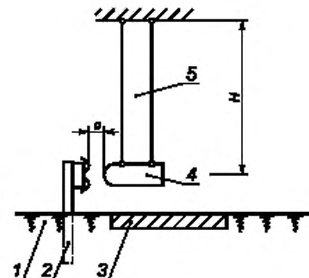
Рисунок 3 — Схема площадки для стеновых ударных испытаний
