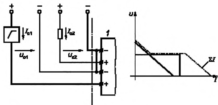
d — Параллельное подключение со сложением значений тока и, возможно, напряжения
