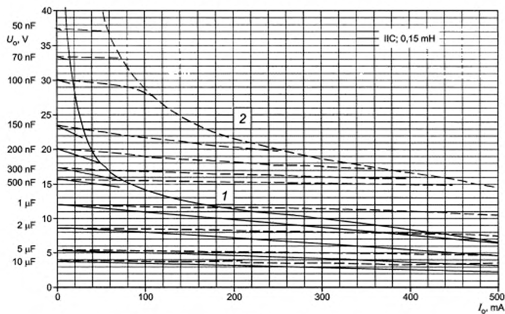
Рисунок С.7в — Диаграмма для 0,15 мГн (продолжение)
