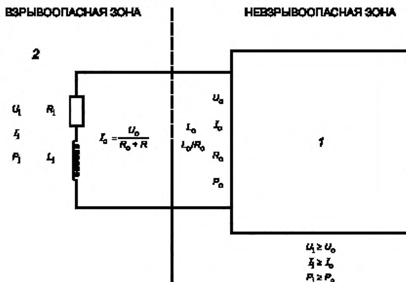
Рисунок D.1 — Типовая индуктивная цепь
