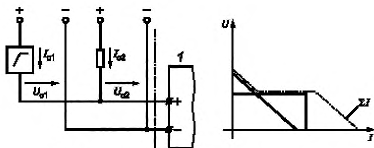
с — Параллельное подключение со сложением значений тока
