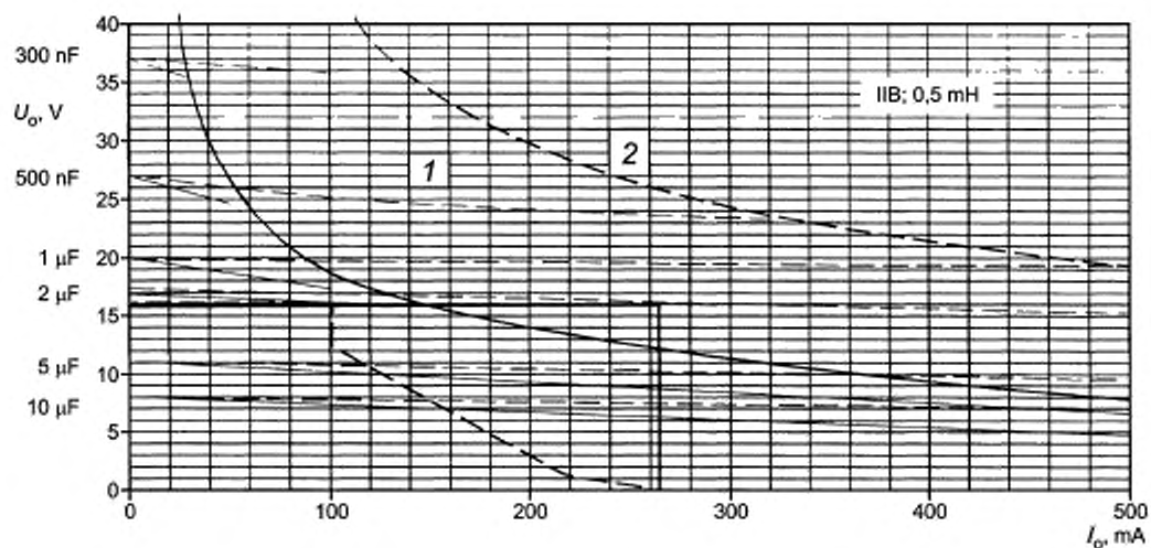
Рисунок С.6а — Сложение тока
