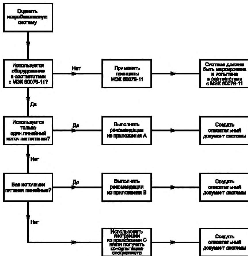
Рисунок 1 — Оценка систем
