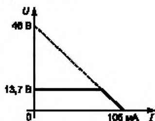
а - выходная характеристика
