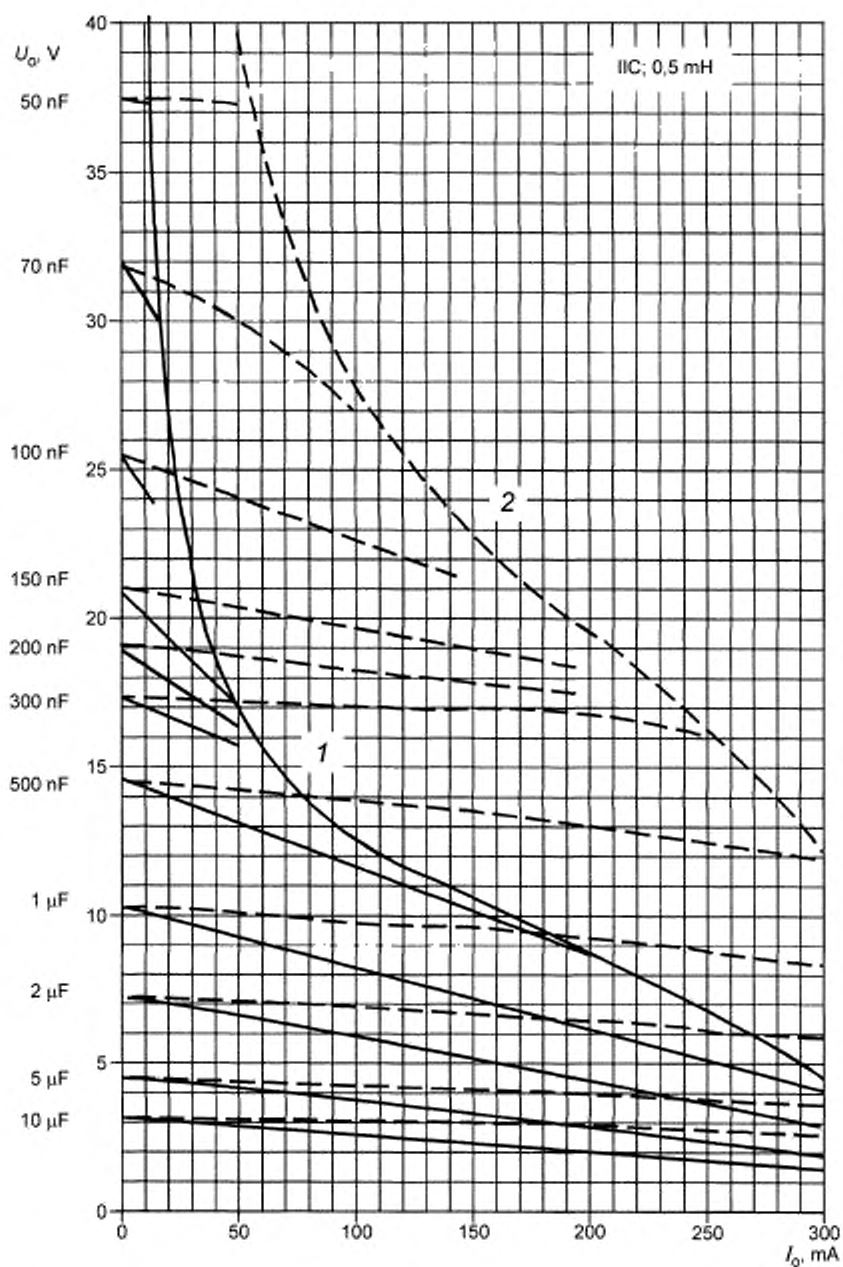
Рисунок С.7в — Диаграмма для 0,5 мГн
