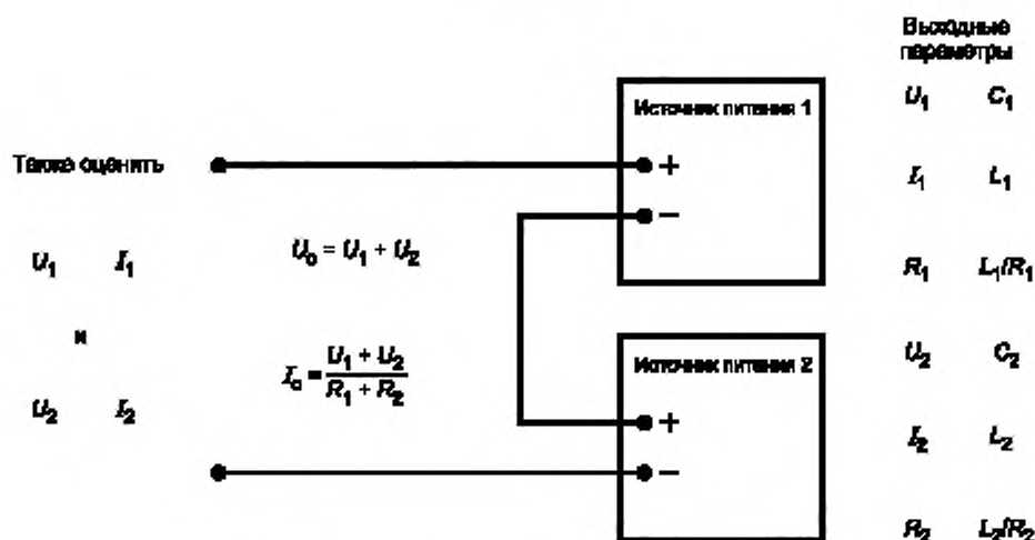
Рисунок В.1 — Последовательно подключенные источники питания
