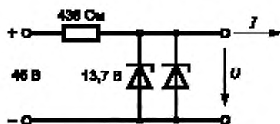
б - эквивалентная цепь
