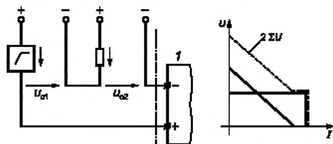
а — Последовательное подключение со сложением значений напряжения
