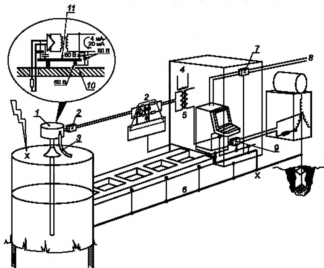
1 — преобразователь; 2 — ограничитель перенапряжений; 3 — заземляющая перемычка; 4 — сетевое питание; 5 — гальванический разьединитель; 6 — эквипотенциальное соединение; 7 — подавитель сигналов; 8 — канал передачи данных; 9 — сетевой фильтр-подавитель; 10 — обшивка резервуара; 11 — корпус прибора
