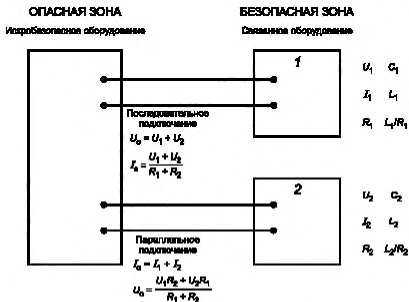
Рисунок В.3 — Произвольно подключенные источники питания
