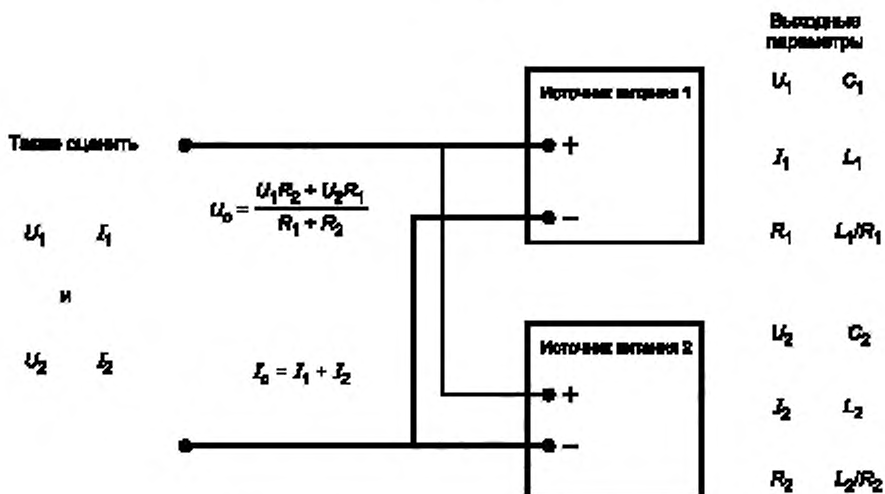
Рисунок В.2 — Параллельно подключенные источники питания
