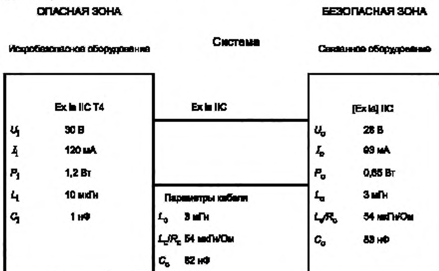
Рисунок А.1 — Соединение искробезопасного оборудования и связанного оборудования
