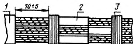
1 — электрический соединитель; 2 — бирка; 3 — бандаж
