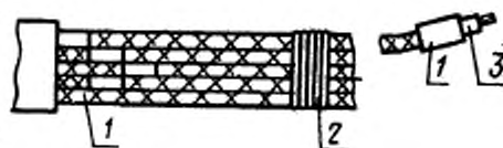
1 — бирки; 2 — бандаж; 3 — наконечник
