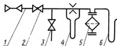
1 — воздушная линия; 2 — проходной кран; 3 — зажим; 4 — реометр с диафрагмой; 5 — испытуемый фильтр-поглотитель; 6 — U-образный мановакуумметр
