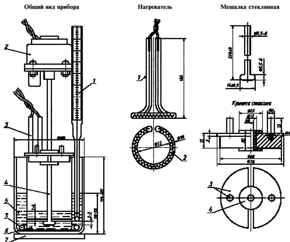
1 — электроконтактный термометр; 2 — электродвигатель; 3 — нагреватель; 4 — мешалка; 5 — водяная баня; 6 — стакан для перемешивания смеси масла и раствора едкого натра; 7 — асбест
