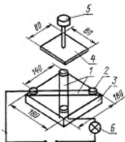
1—образцы провода; 2—цилиндрические штыри; 3—нижняя пластина; 4—верхняя пластина; 5—груз; 6—сигнальная лампа.
