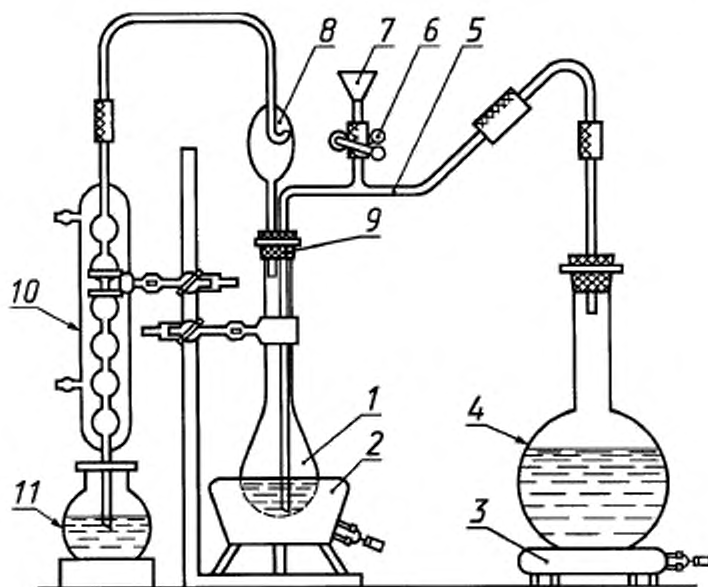
1 — колба Кьельдаля; 2 — колбонагреватель; 3 — электролитка; 4 — паробразователь; 5 — соединительная трубка; 6 — зажим; 7 — воронка; 8 — каплеуловитель; 9 — пробка; 10 — холодильник; 11 — приемная колба
