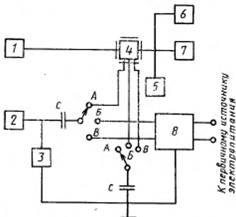
1, 2 — высокочастотные генераторы сигналов; 3 — нагрузка генератора сигналов с сопротивлением R_n = 50 (75) Ом; 4 — приемник; 5 — испытательная нагрузка приемника; 6 — низкочастотный вольтметр переменного тока; 7 — измеритель нелинейных искажений; 8 — фильтр питания; C — конденсаторы (1000 пФ); A — подключение к линии управления; B и B — подключение к линии электропитания
