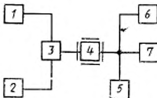
1, 2 — высокочастотные генераторы сигналов; 3 — согласующее устройство 1-го типа; 4 — приемник; 5 — испытательная нагрузка приемника; 6 — низкочастотный вольтметр; 7 — измеритель нелинейных искажений
