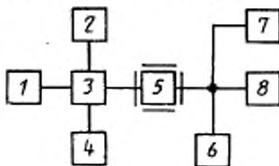
1, 2, 4 — высокочастотные генераторы сигналов; 3 — согласующее устройство 2-го типа; 5 — приемник; 6 — испытательная нагрузка приемника; 7 — низкочастотный вольтметр переменного тока; 8 — измеритель нелинейных искажений
