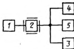
1 — высокочастотный генератор сигналов; 2 — приемник; 3 — испытательная нагрузка приемника; 4 — низкочастотный вольтметр; 5 — измеритель нелинейных искажений
