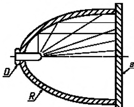
D — излучатель; R — рефлектор; B — фотоприемник
