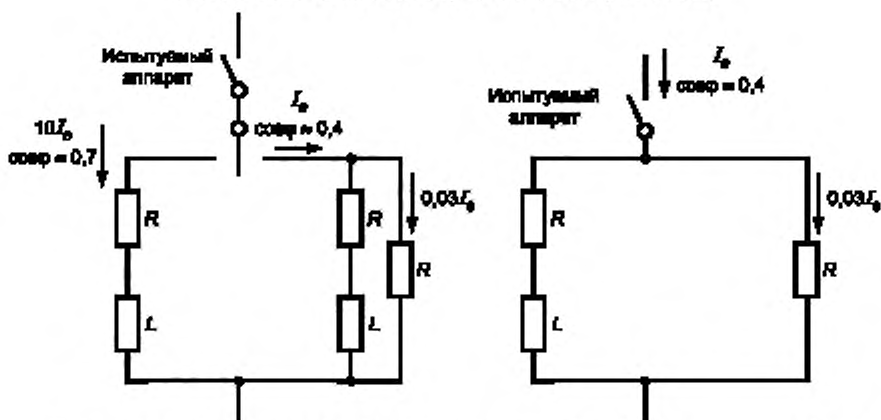
Рисунок С.1 — Полная схема (см. С.3.2.1)
