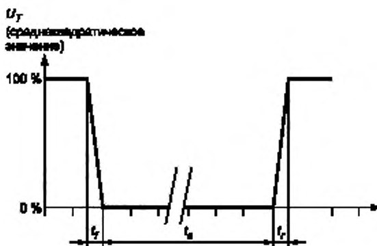
Рисунок 2 — Кратковременное прерывание напряжения
