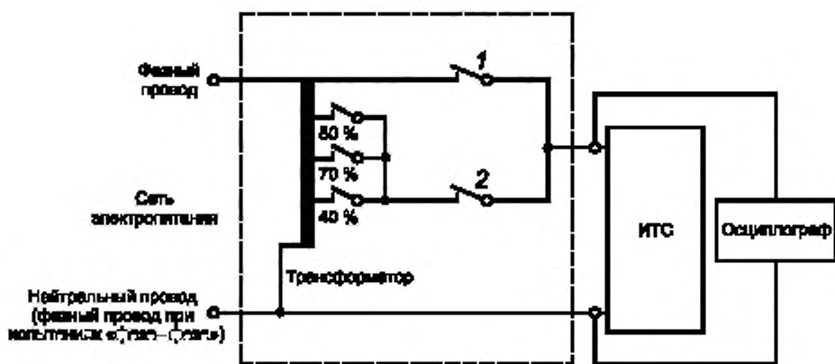
в) Схема испытаний с использованием трансформатора с отводами и переключателей
