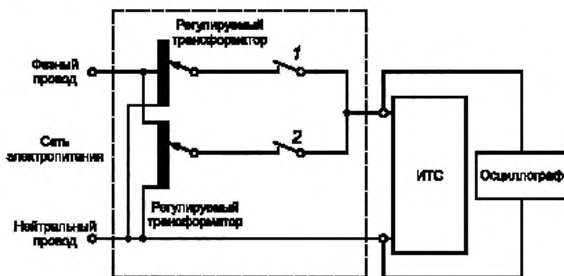
1, 2 — попеременно коммутируемые переключатели
