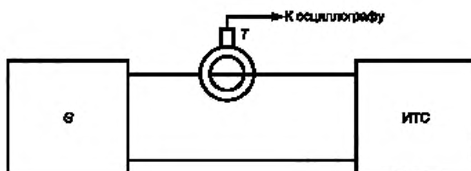
Рисунок А.2 — Схема измерения пикового значения потребляемого тока ИТС
