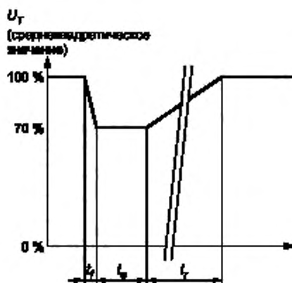
Рисунок 3 — Изменение напряжения
