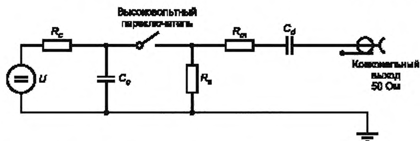
Рисунок 1 — Упрощенная схема ИГ
