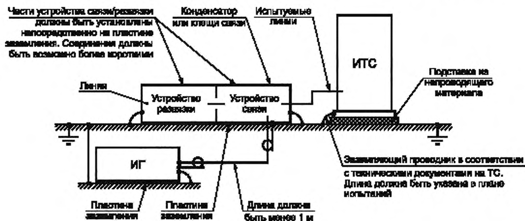
Рисунок 6 — Схема испытаний ТС на устойчивость к НИП
